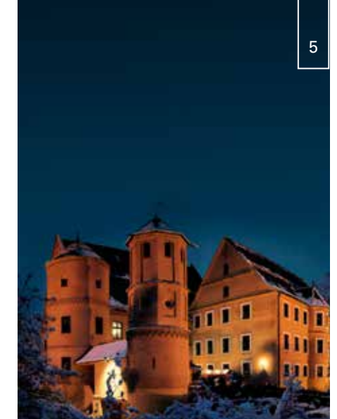
Sanierung Schloss Wertingen (14. Jh.): Die Klimadecke temperiert das Schloss äußerst energieeffizient, obwohl kein Vollwärmeschutz vorhanden ist. Selbst bei frostigen -16 °C Außentemperatur genügen 39 °C Vorlauftemperatur für ein behagliches Raumklima bei 22 °C.
